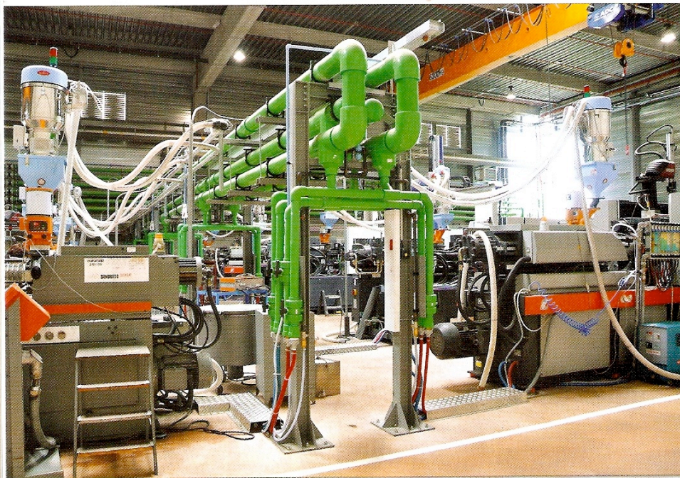
Le système de récupération des calories générées par le refroidissement des presses à injecter permet de stocker l'énergie pour chauffer les bâtiments l'hiver.
